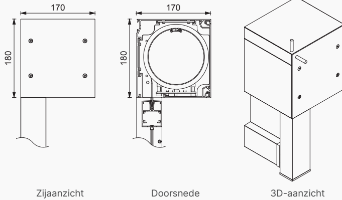
Zijaanzicht
