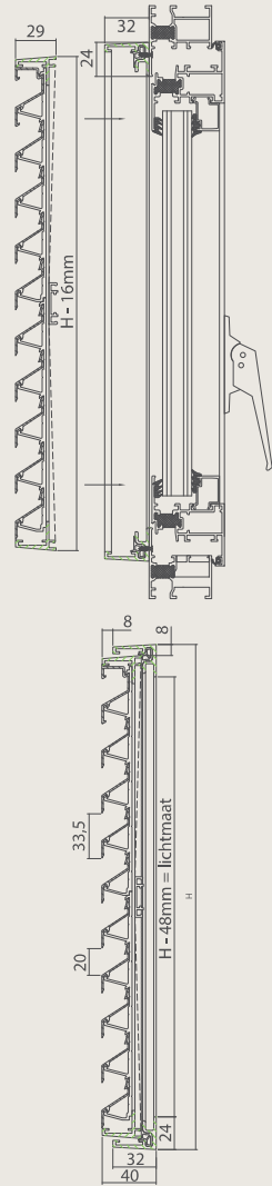
Doorsnedetekening
